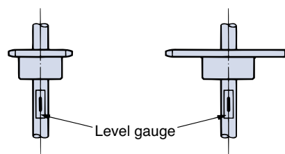
Fig. 15 Horizontal precision
